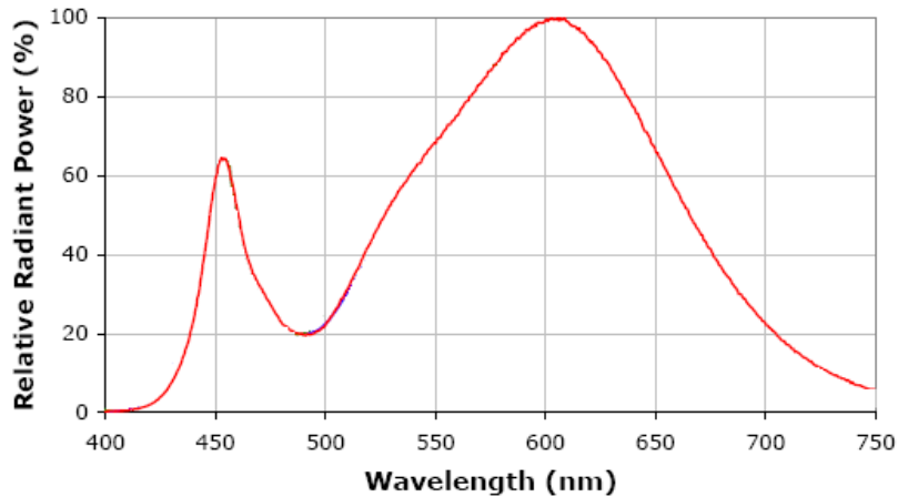
暖白光光谱图
